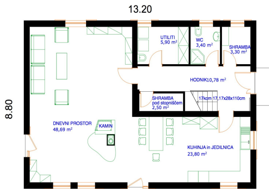
PRITLIČJE
